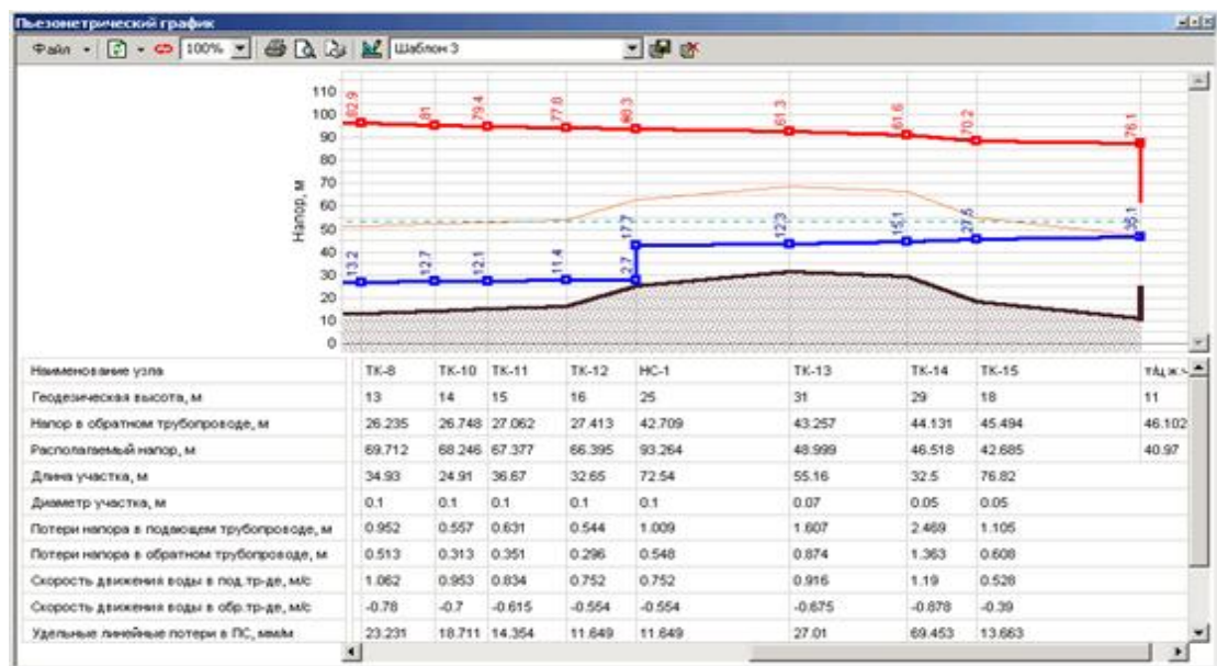
Рисунок 2.14 - Пьезометрический график
