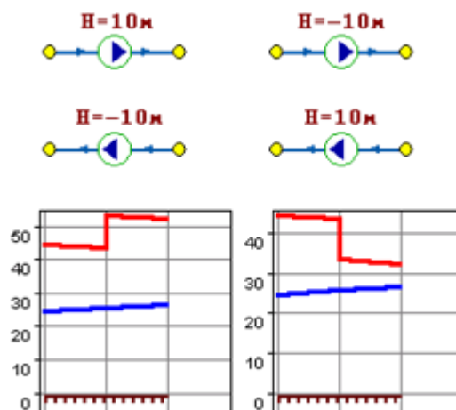
Рисунок 2.8 - Пьезометрические графики
