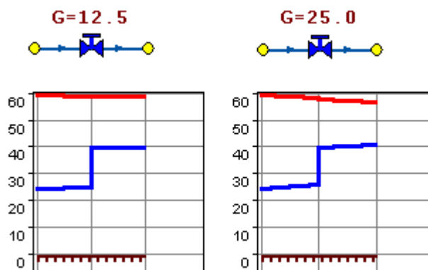
Рисунок 2.12 - Регулятор давления
